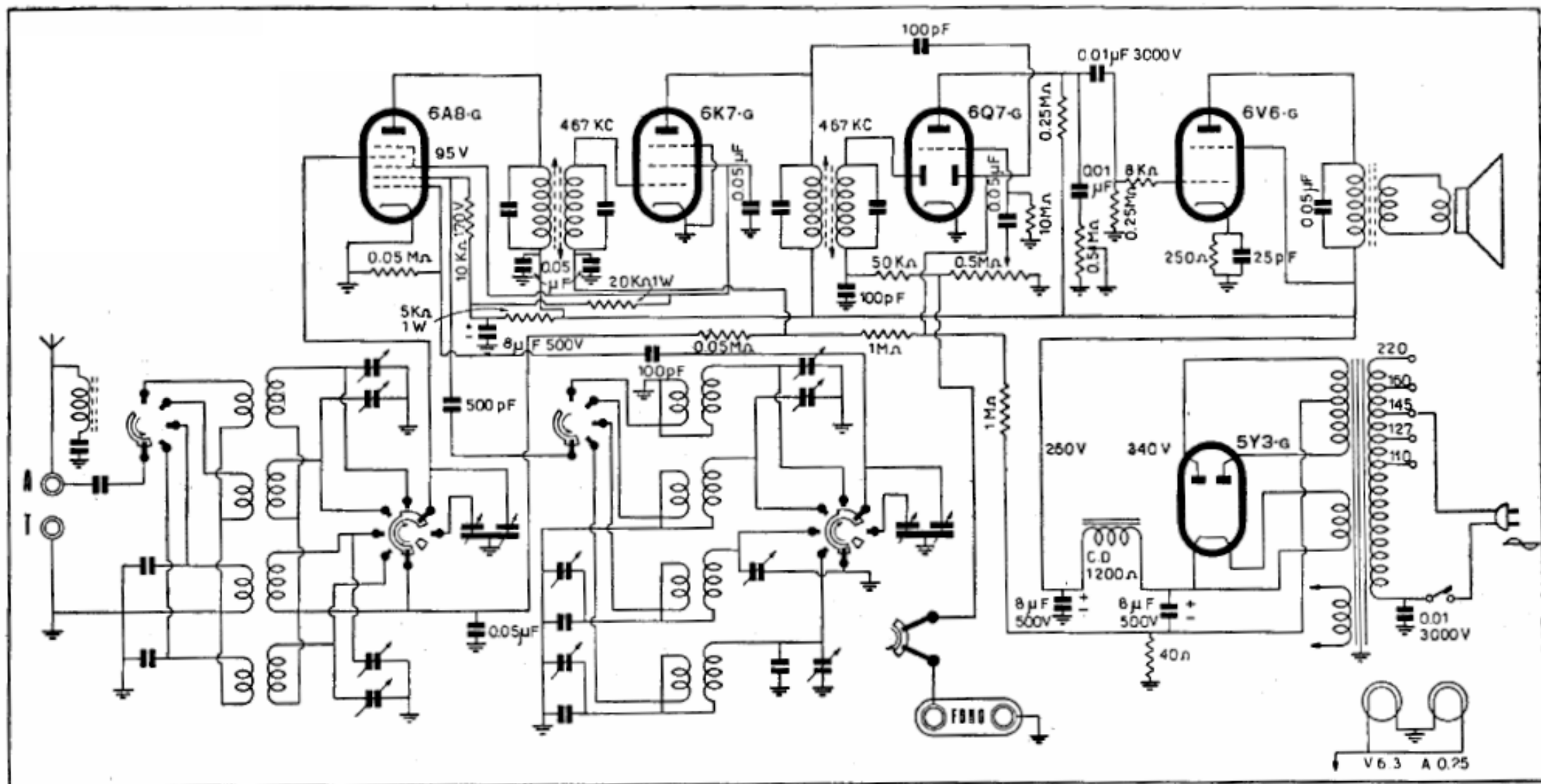
IRRADIO - Mod. 58 - Quattro gamme d'onda. Media frequenza 467 kc. Potenza d'uscita 4 W. Consumo 60 W.
